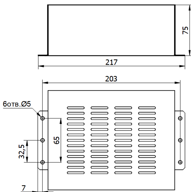
Рисунок 1 - Габаритные размеры защитного кожуха
